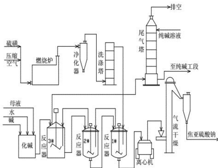
图2.2-3 焦亚硫酸钠生产工艺图
