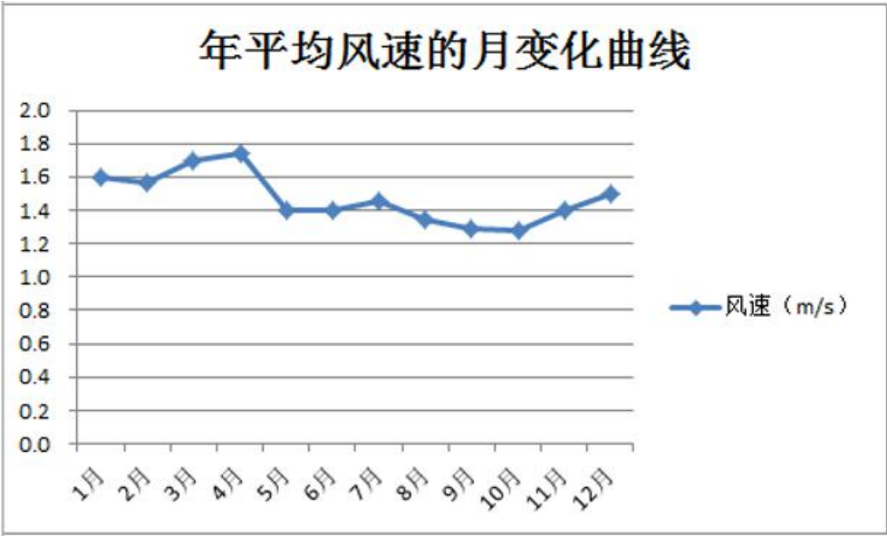
图 4.2-2 年平均风速月变化曲线
