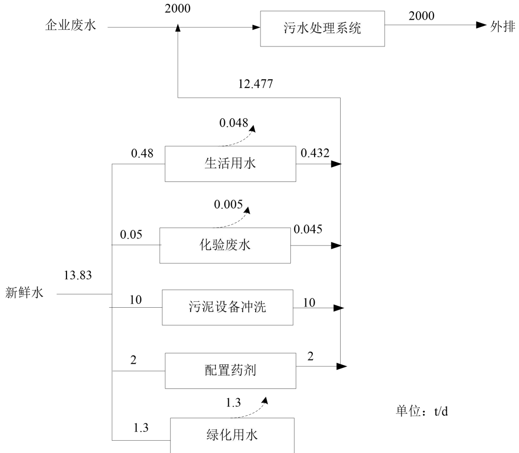
图 2.4-1 水平衡图
