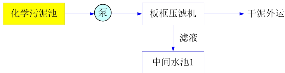
图2.2-8 化学污泥处理系统工艺流程
