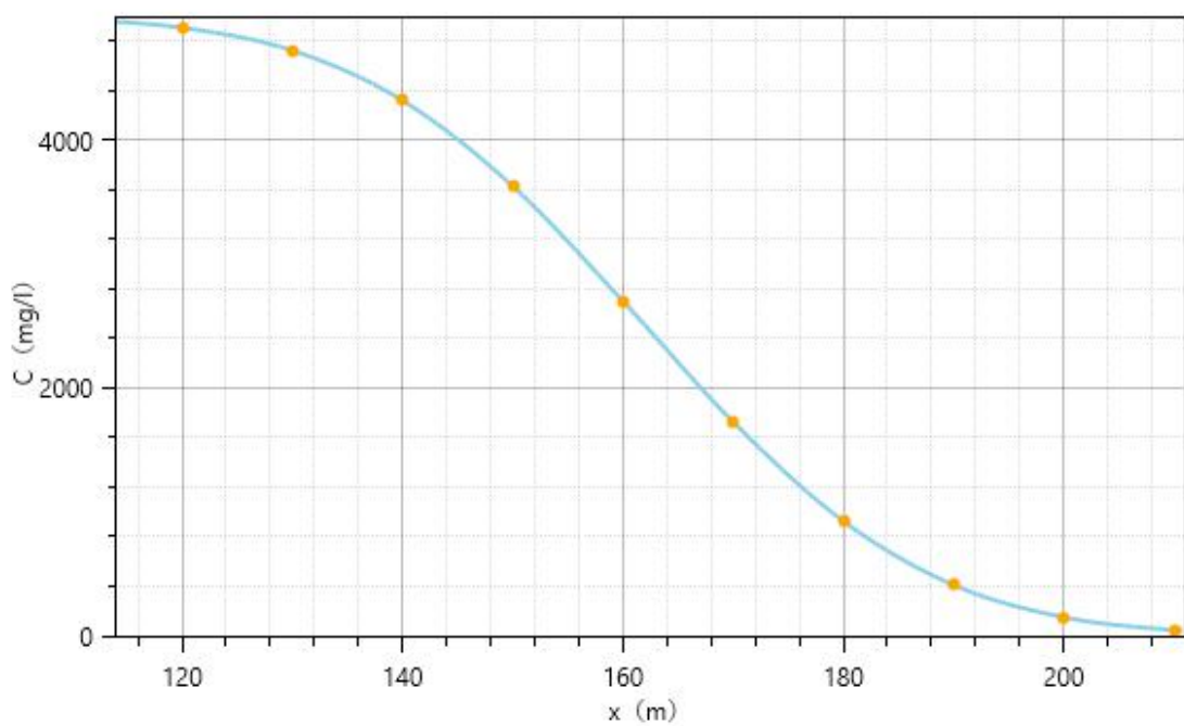
图 4.2-5 (2) 渗漏 1000 天 COD 污染物不同距离浓度预测曲线
