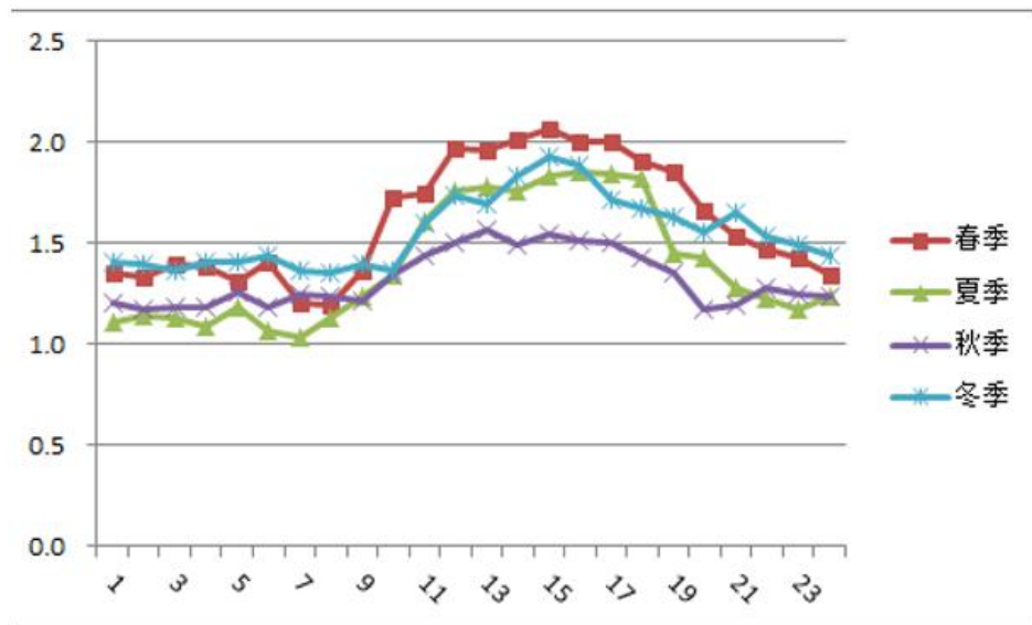
图4.2-3 季小时平均风速日变化情况曲线
